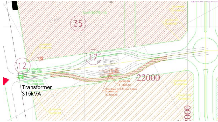
شکل ۱: محل قرارگیری ترانسفورمر 315 kVA
