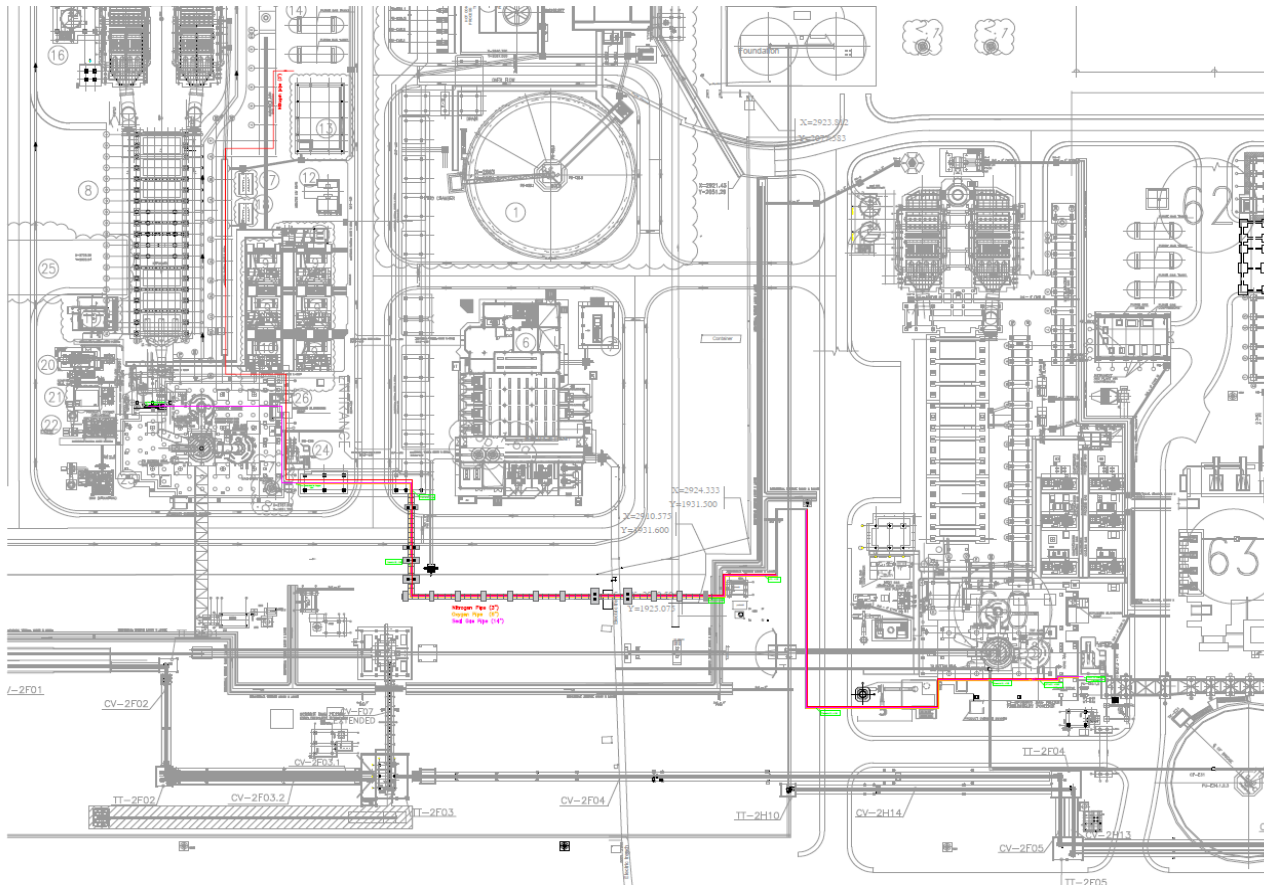
شکل ۱ مسیر اجرایی پایپینگ لاین های ازت و اکسیژن و سیل واحد طوبی
