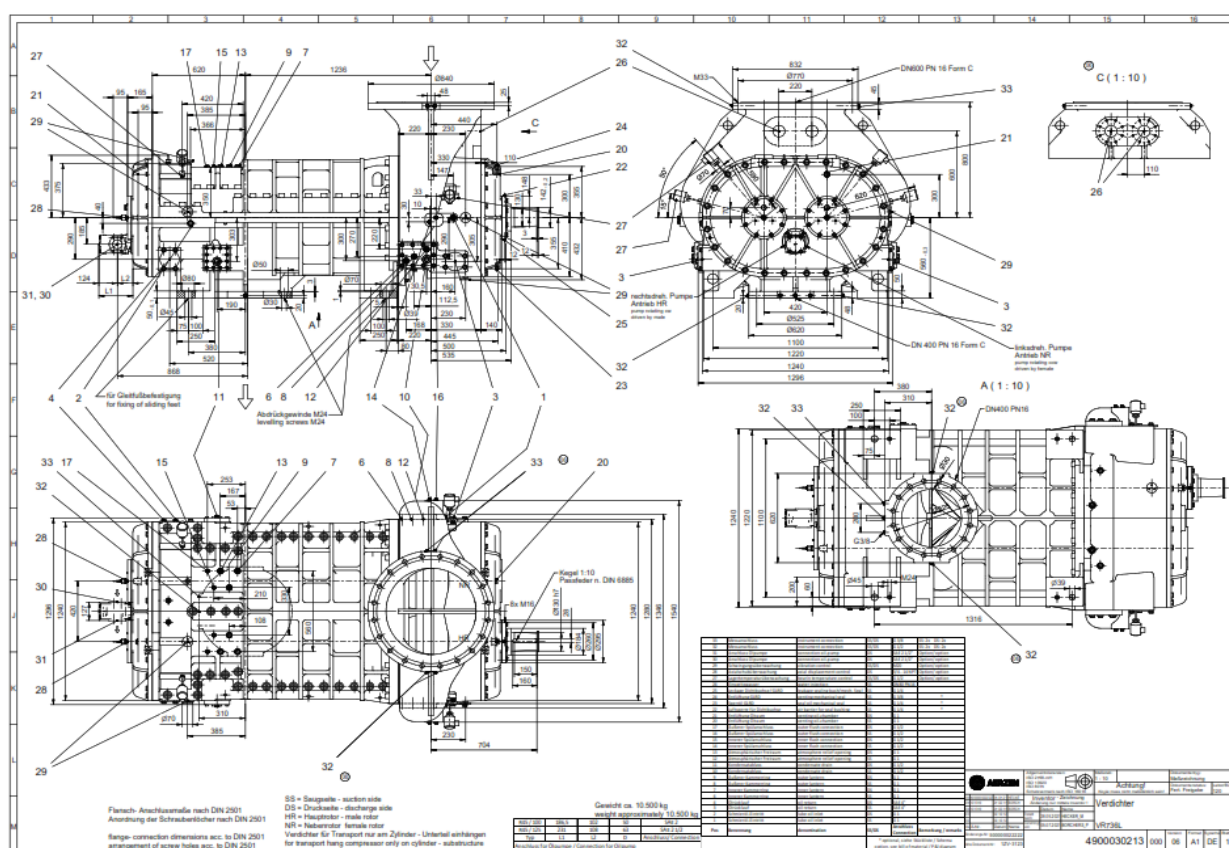
شکل ۱: نقشه ی ابعادی کمپرسور اسکرو
