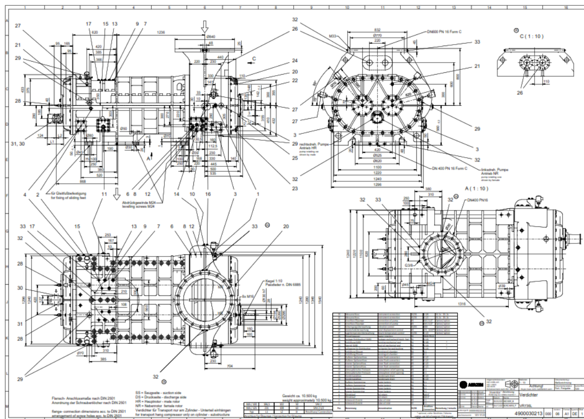
شکل ۱: نقشه‌ی ابعادی کمپرسور اسکرو
