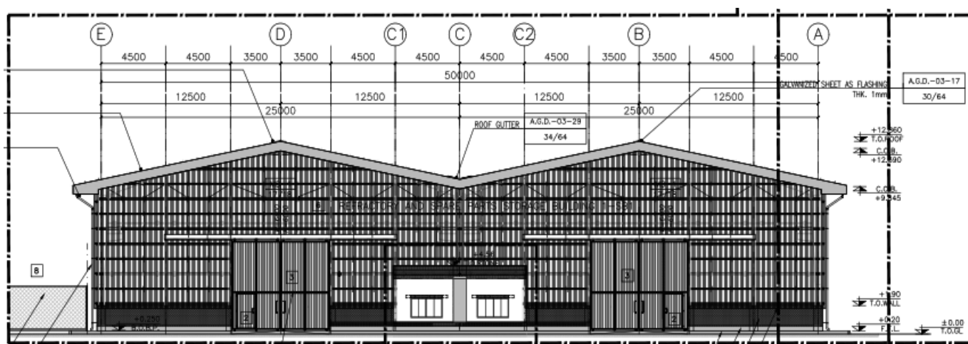
شکل ۱: انبار نسوز شماره ۱
